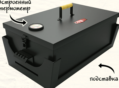
Коптильня двухъярусная с подставкой размер: 54x31x45 см в комплекте: 2 решетки, поддон для стекания жира материал: сталь 1,5 мм встроенный термометр
