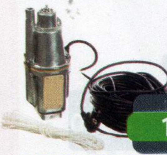
НАСОС ВИБРАЦИОННЫЙ МАЛЫШ-М , 10м, верх.забор, 1500л/ч, 240Вт
